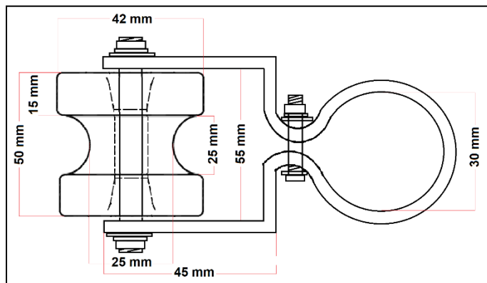
Ilustración 2. Aislador cerámico con soporte de 1 ½ pulgadas
